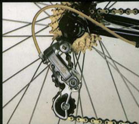
Shimano 105 rear derailleur.
